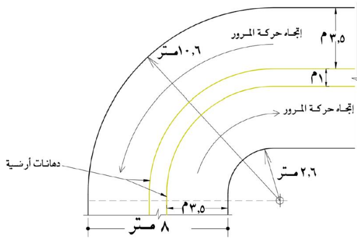
(٥) الحد الأدنى للمنحنى للسير باتجاهين في المواقف السطحية
