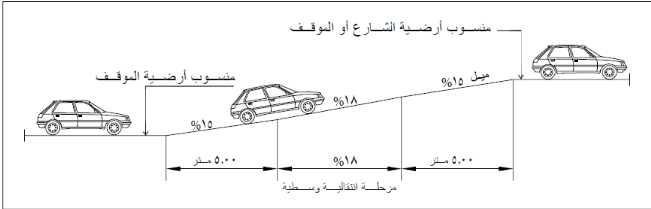
شكل (٧) المنحدر المستقيم ومراحله الانتقالية
