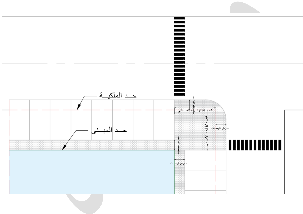
شكل (٨) يوضح بداية أول موقف في التقاطعات
