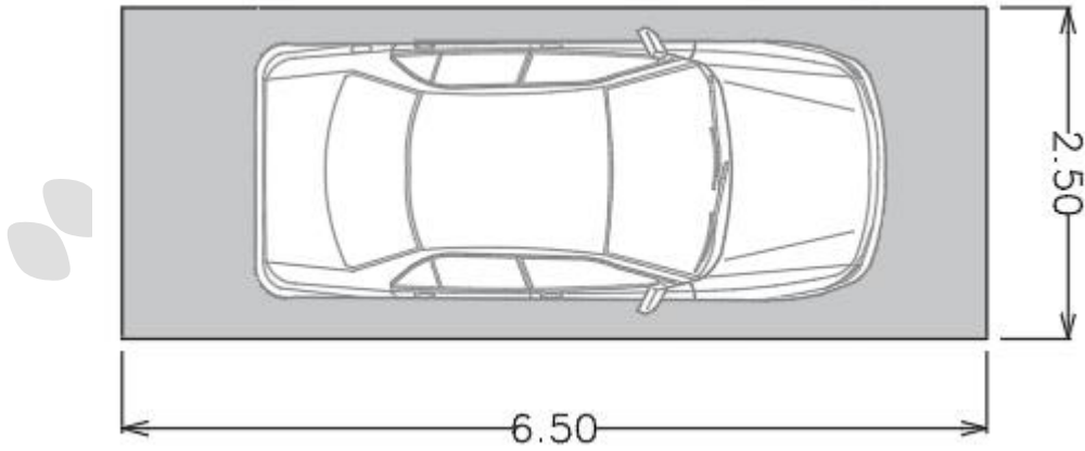
شكل (١) الحد الأدنى لأبعاد الموقف الموازي (الطولي) للطريق
